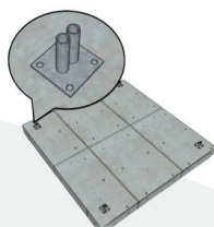
Etape 3 : Placement des rehausses
