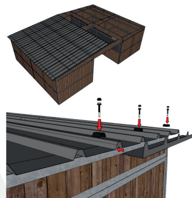
Etape 4 : Placement de la toiture
